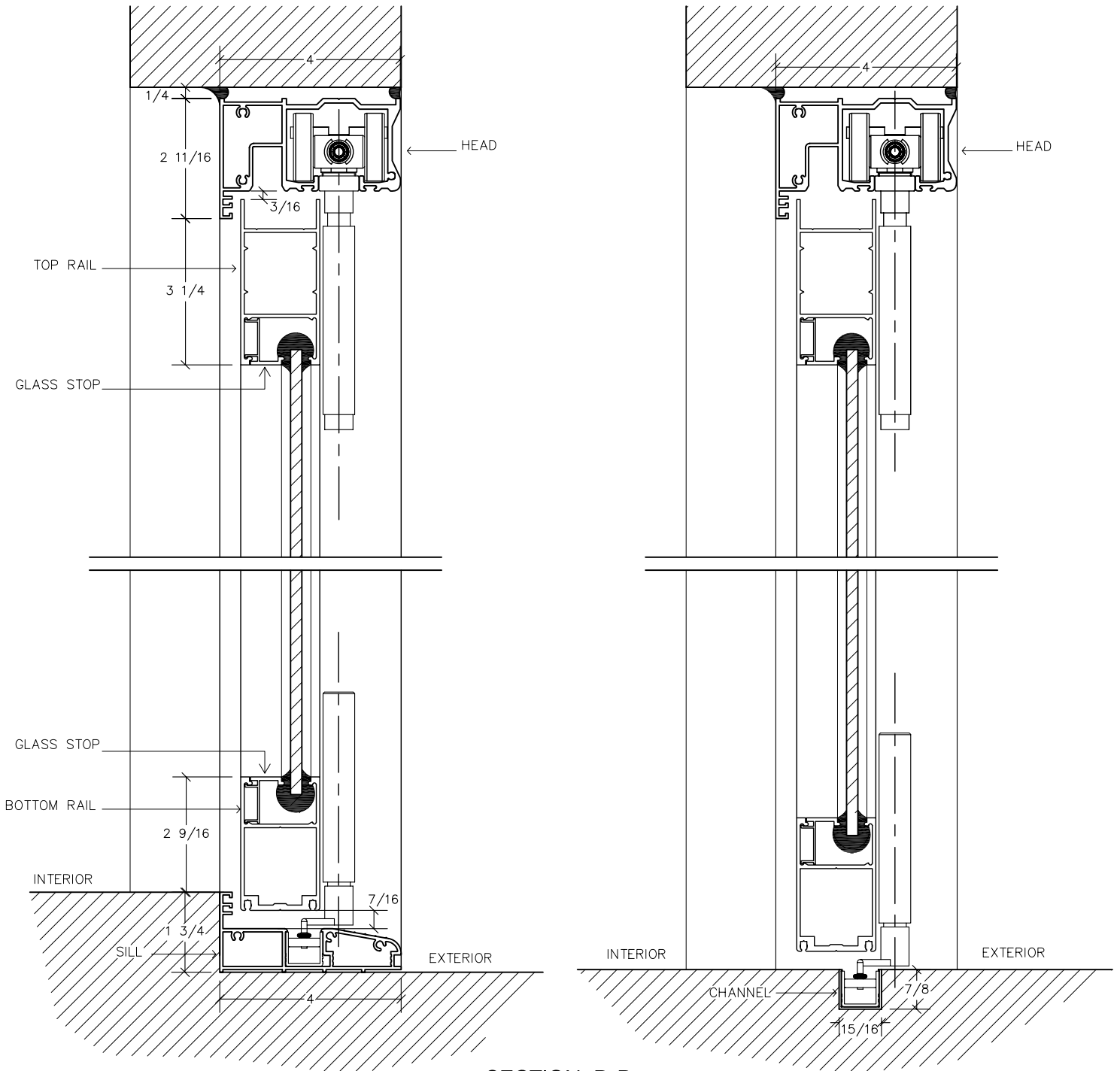
SECTION D-D
