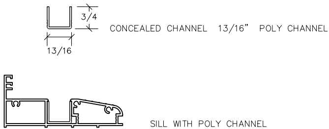
SECTION D-D
