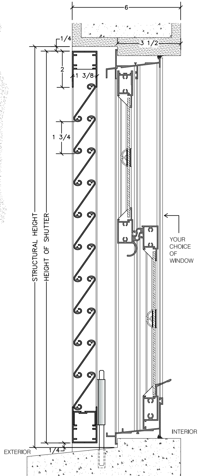
SECTION A-A
